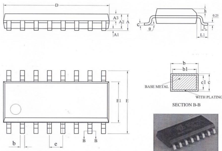
图 11-1 PAN3020 芯片 SOP16 封装图
