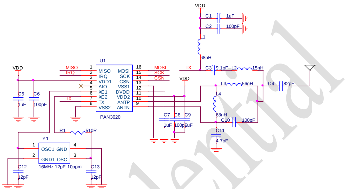
图 10-1 PAN3020 SOP16 433MHz 频段应用电路
