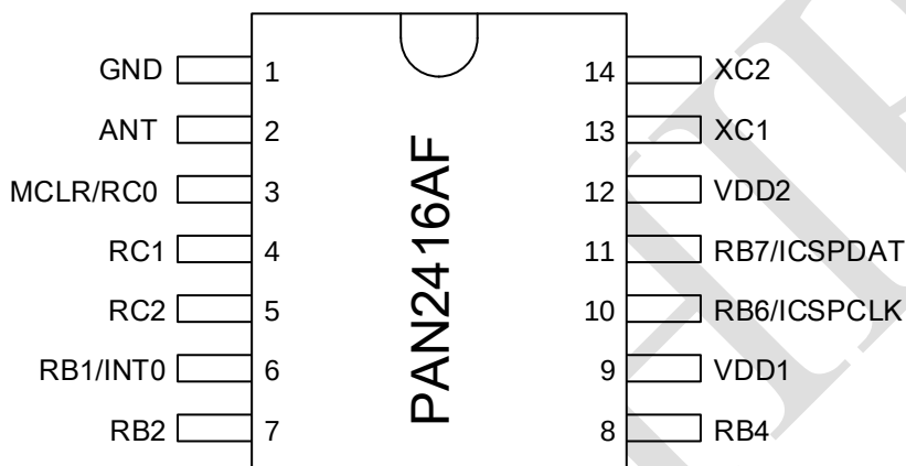
图 3-1 PAN2416AF 芯片引脚图
