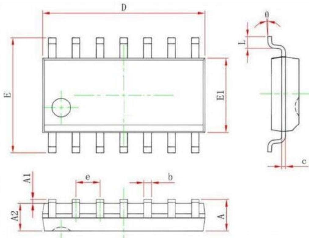
图 22-1 PAN2416AF 封装图（SOP14）
