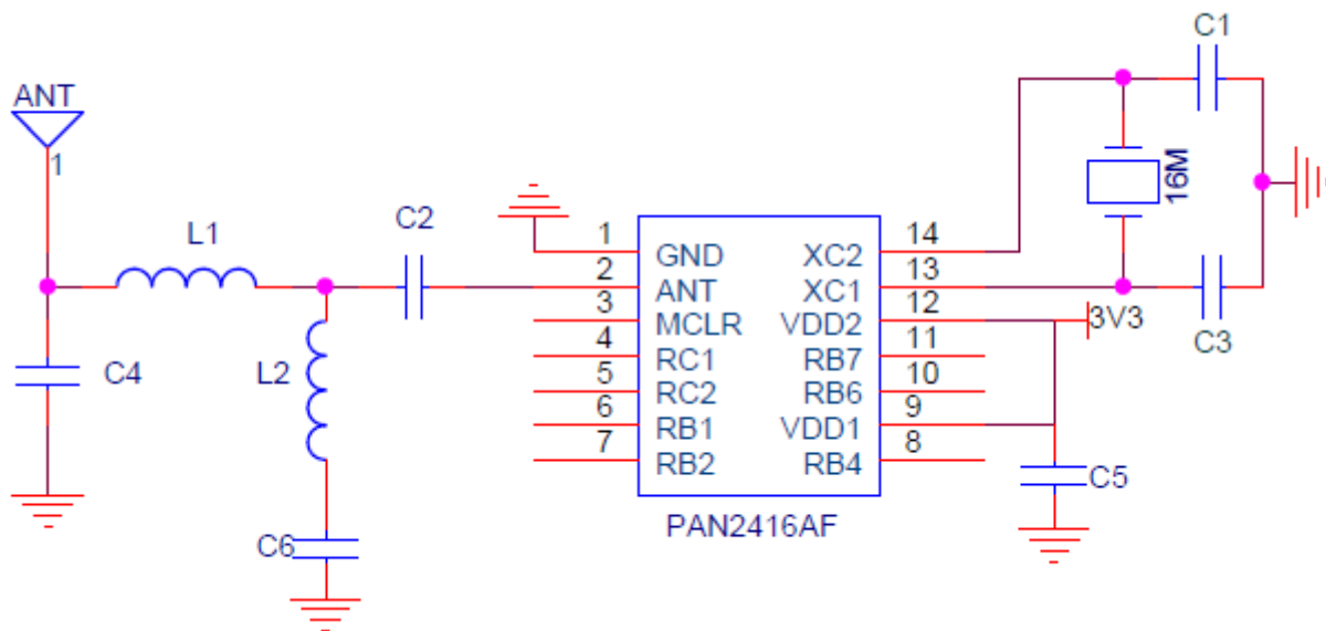
图 21-1 PAN2416AF 的应用电路
