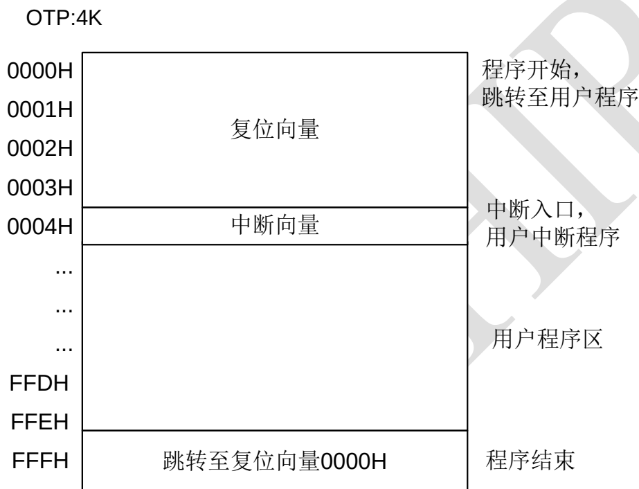
图 11-1 PAN2416AF 芯片程序存储器空间
