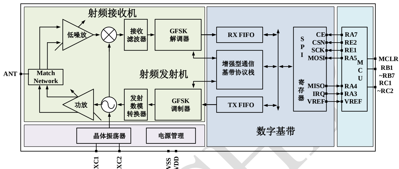
图 2-1 PAN2416AF 芯片系统结构方框图
